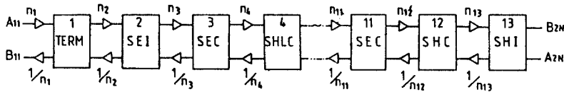
그림 9 스케일된 WDF의 블록선도(Dual-2 회로망) Block diagram of scaled WDF(Dual-2 network).
