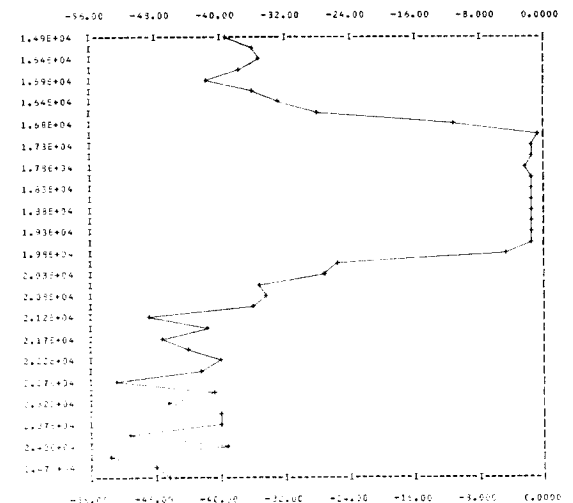
그림 11 스케일된 WDF의 주파수 응답(16비트) Frequency response of scaled WDF(16 bit).
