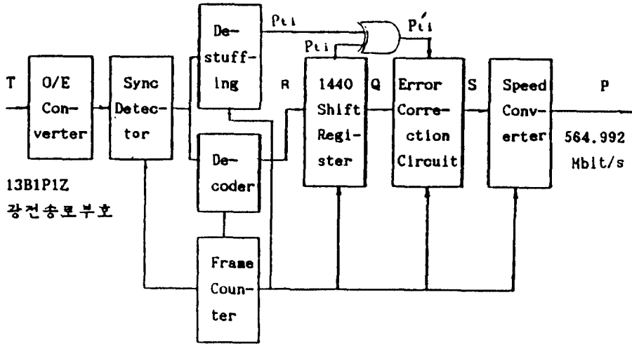
그림 5. 단국중계장치 수신단의 시스템 블럭도 Fig. 5. System block diagram at receiver of TRS
