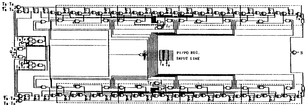
그림 7. 에러교정회로 Fig. 7. Error Correction Circuit
