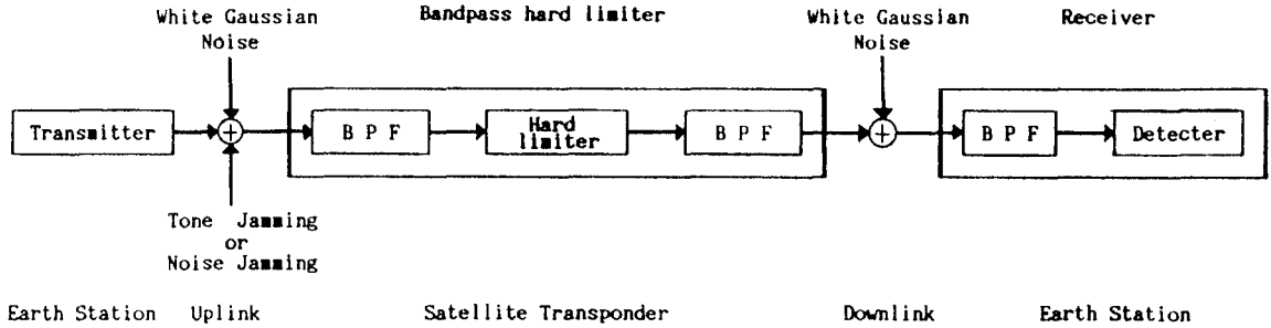
그림 1. 하드러미터형 중계기를 채용한 위성통신 시스템 Satellite communication system with hard limiter type transponder.
