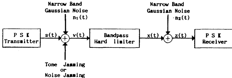
그림 2. 하드러미터형 중계기를 채용한 PSK 위성통신 시스템의 해석모델 Analysis model of PSK satellite communication system with hard limiter type transponder.
