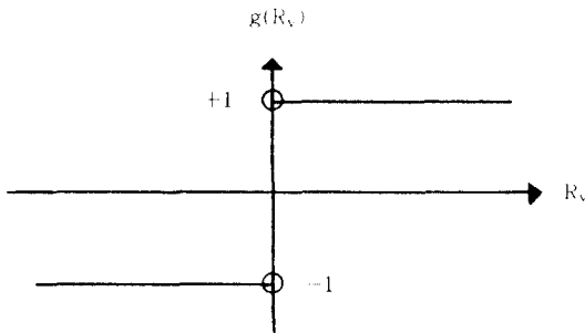
그림 3. 하드러미터의 입력-대 출력 특성 Input-output characteristic of hard limiter.
