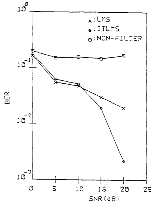
그림 19. LMS 및 ITLMS 알고리즘을 사용한 DS 대역 확산 통신 시스템의 비트 에러율
