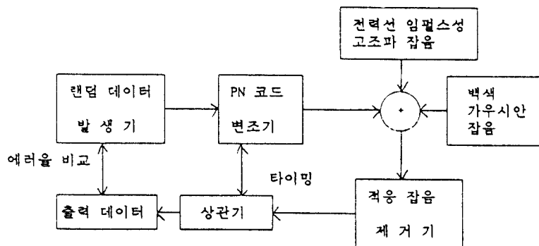
그림 7. 시뮬레이션을 위한 시스템 구성도
