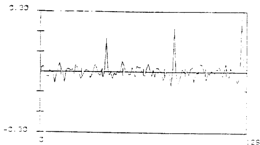
그림 13. LMS 알고리즘을 사용한 경우의 필터 계수
