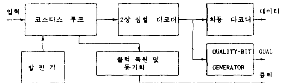
그림 3. 기존 라디오 데이터 복원기의 구성도. Fig. 3. Block diagram of already existing radio data demodulator.
