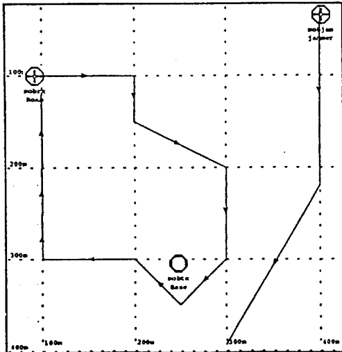
그림 5-18. 수신기와 jammer의 궤적도. Fig.5-18. trajectory of receiver & jammer.
