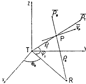
그림 2-5. bistatic 레이더의 추적. Fig.2-5. bistatic radar measurement.
