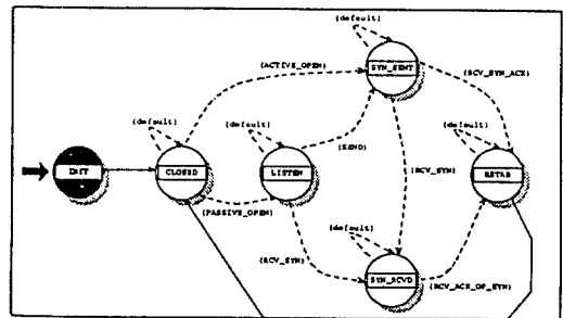
그림 5-10. tcp 블럭의 상태 전이도. Fig.5-10. state diagram of tcp node.
