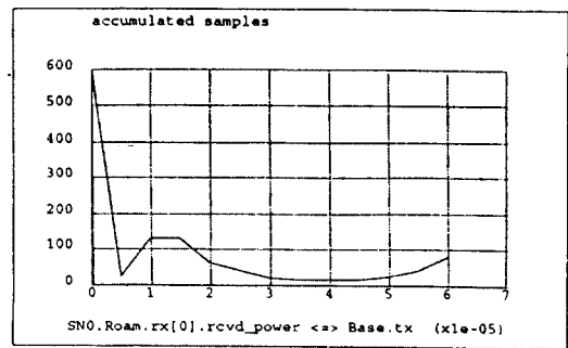
그림 5-24. 신호전력의 히스토그램. Fig.5-24. histogram of rcved signal.
