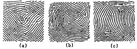
그림 7. 오분류된 부분패턴
