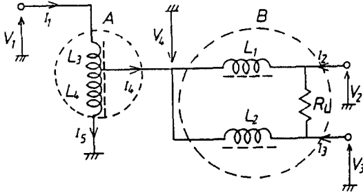
그림 3. 입력단이 보상된 윌킨슨형 신호분배기 Fig. 3. Wilkinson type power divider Compensated at Input Port
