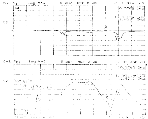
그림 12. OFF 상태에서 측정된 S_{11} 과 S_{21} 특성. Fig. 12. S_{11} and S_{21} at OFF-state.
