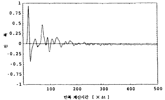
그림 3. 반복 계산시간에 따른 전압파형.
