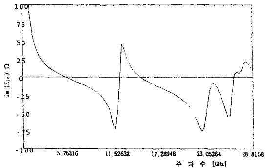
그림 5. 원형편파 마이크로스트립 안테나 급진점 F에서의 입력임피던스.
