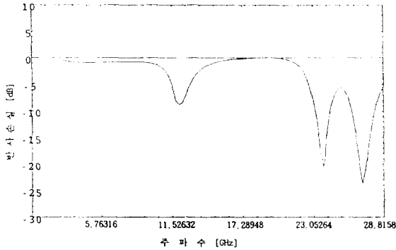
그림 4. 원형편파 마이크로스트립 안테나의 급진점 F에서의 반사손실.
