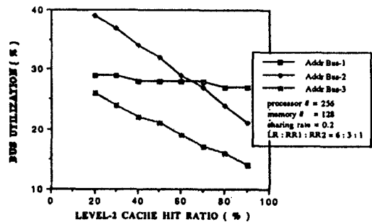
그림 5-8. 레벨-2 캐시 적중률에 따른 어드레스 버스의 사용률.
