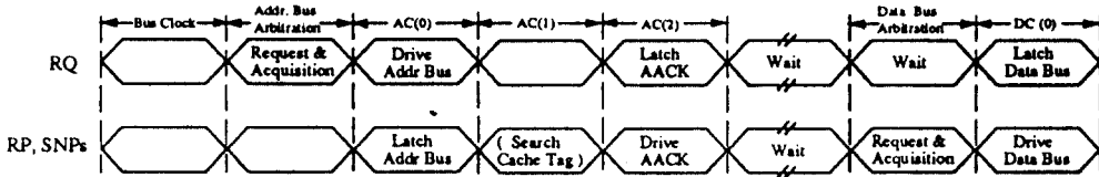
그림 5-4. RFR 동작 순서.
