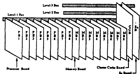
그림 3-2. 3-레벨 계층 클러스터 구조에서의 클러스터 구성도.
