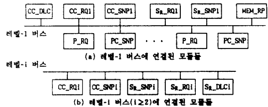
그림 5-2. 각 레벨 버스의 기능 블록.
