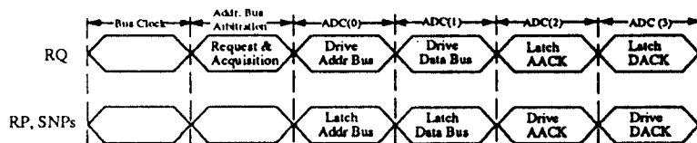
그림 5-6. WRB 동작 순서.
