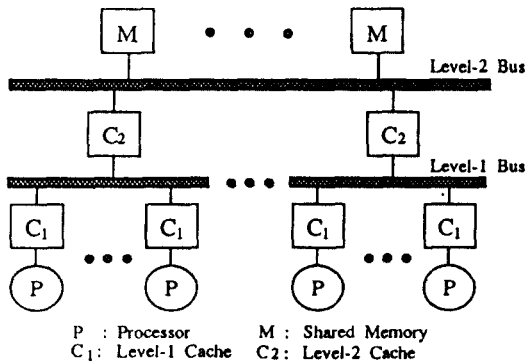
그림 2-1. Wilson의 캐시 버스/캐쉬 구조.
