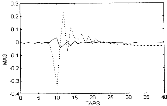
— 정상적인 통화 상태에서의 반향 경로 응답 ..... 2선/4선 변환 회로에서의 임피던스 비 매칭시 반향 경로 응답
