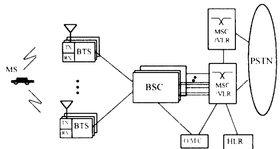
그림 1. CDMA 이동 통신 시스템 구조 Fig. 1 Architecture of CDMA mobile communication system.
