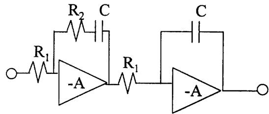
그림 2 적분기 구성도
