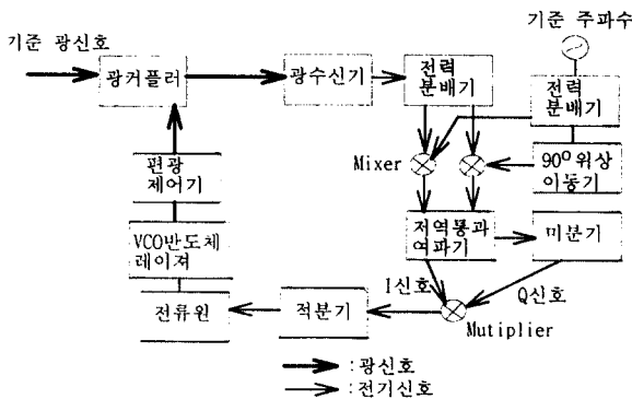
그림 1 광주파수 동기화장치 구성도
