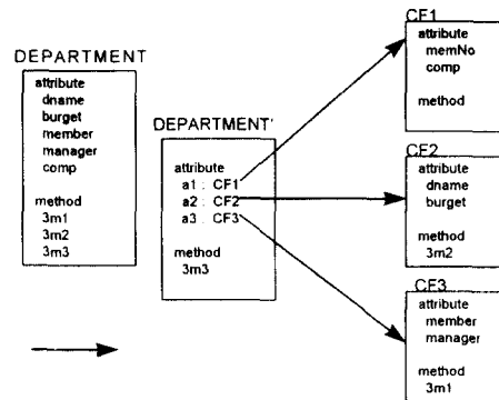
그림 10. DEPARTMENT 클래스의 변형
