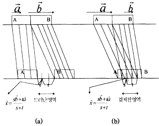
그림 3. 움직임 보상 보간 기법 (3) (a) 드러난 영역에 대한 보상 (b) 겹쳐진 영역에 대한 보상
