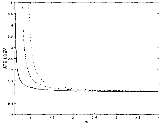
그림 4. ARE_{LS, EV}
