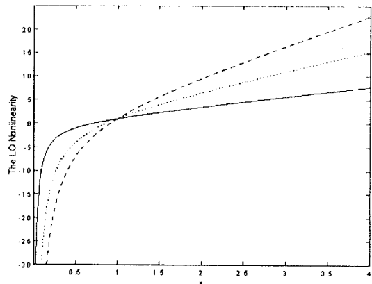
그림 1. \sigma^2=1, m=1 (solid), m=2 (dotted), m=3 (dashed)일 때 국소최적 비선형성
