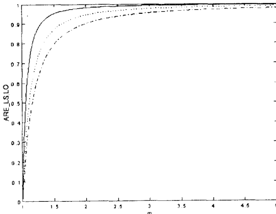
그림 5. ARE_{LS, LO}
