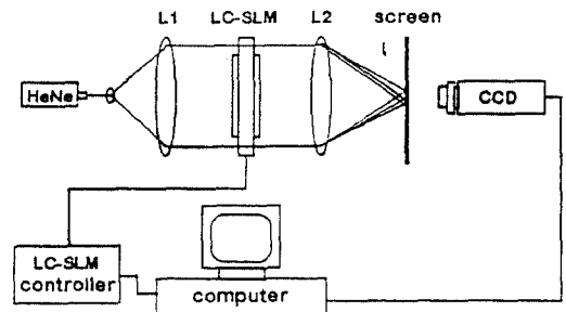
그림 10. SLM을 이용한 빔 패턴 발생장치
