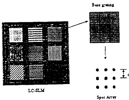
그림 9. SLM에 기록되는 회절격자의 배치도
