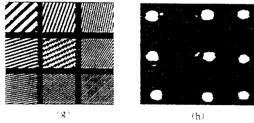
그림 14. SLM에 디스플레이된 격자 배열과 출력평면에서의 연결결과 (a)4개의 격자배열입력 (b)포트 4, 12, 14, 22 출력결과 (c)5개의 격자배열입력 (d)포트 4, 12, 14, 22, 24 출력결과 (e)6개의 격자배열입력 (f)포트 2, 4, 12, 14, 22, 24 출력결과 (g)9개의 격자배열입력 (h)포트 1, 3, 5, 11, 13, 15, 21, 23, 25 출력결과
