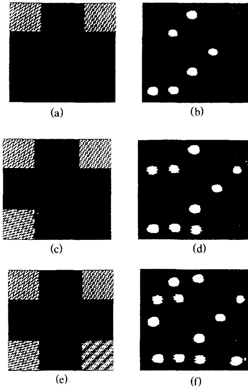
그림 15. 빔 분리와 라우팅을 위한 실험결과 (a)입력빔을 세 개로 분리하는 격자배열 (b)출력포트 4, 5, 8, 12, 19, 23 (c)입력빔을 세 개로 분리하는 격자배열 (d)출력포트 3, 4, 5, 8, 12, 16, 19, 20, 23 (e)입력빔을 세 개로 분리하는 격자배열 (f)출력포트 1, 3, 4, 5, 8, 12, 15, 16, 19, 20, 23, 24
