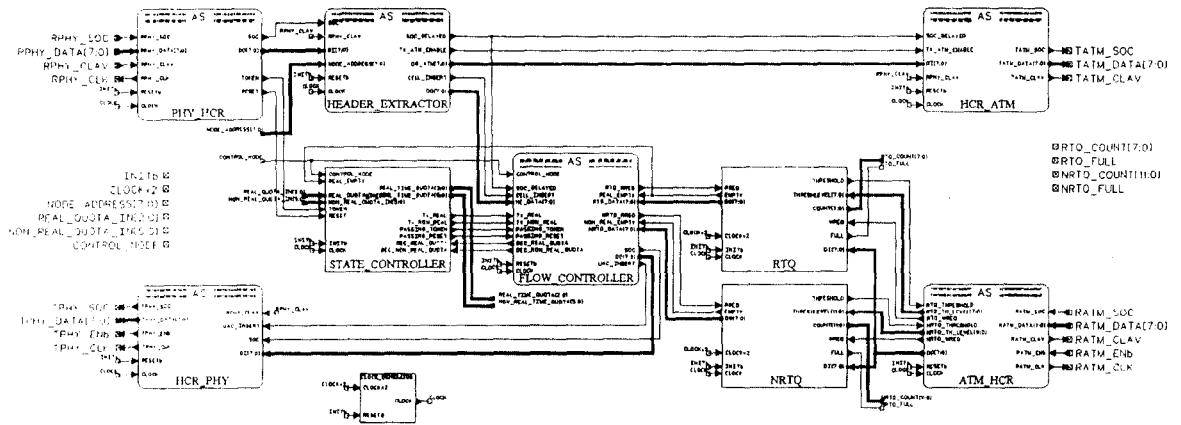
그림 4. 합성된 HCR IC의 Top 블록. Fig 4. Synthesized top block diagram of HCR IC.
