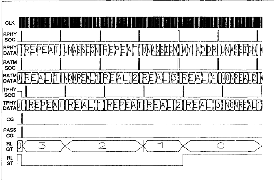
그림 6. 실시간 데이터 전송 결과 파형.
