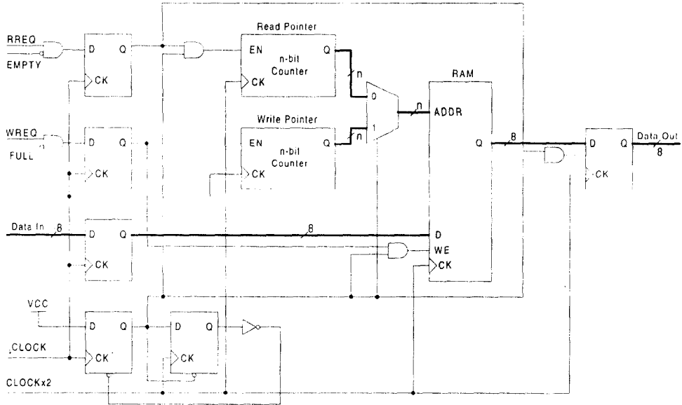
그림 3. 큐의 기본 구조. Fig 3. Basic structure of Queue.
