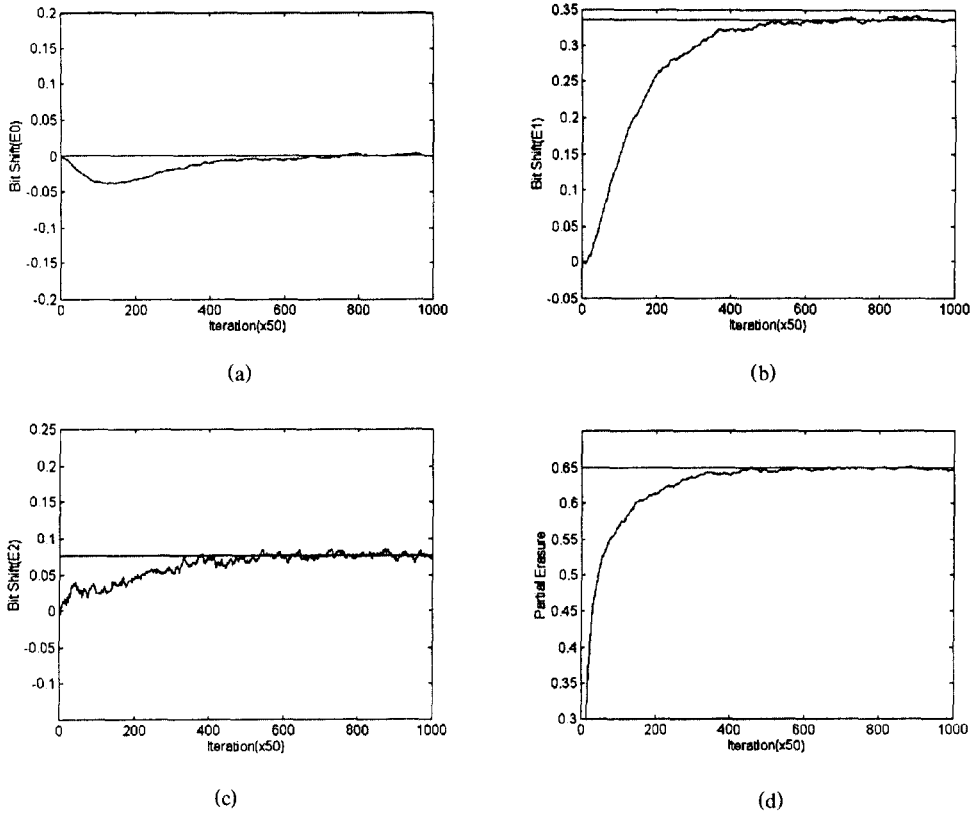
그림 9. 제안된 알고리즘을 사용한 경우 비선형 파라메타의 수렴 특성 (SNR = 20dB)
