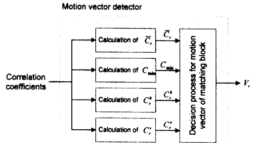
그림 12. 매칭 블록의 움직임 벡터 검출기 Fig. 12. Motion vector detector of matching blocks
