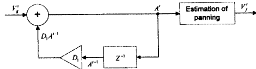
그림 13. 의도적인 패닝의 추정 Fig. 13. Estimation of intentional panning
