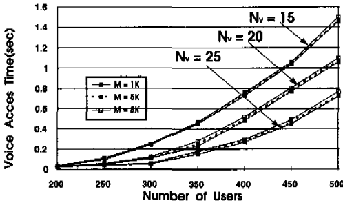
그림 5. D-TDMA 프로토콜에서 음성역세스시간
