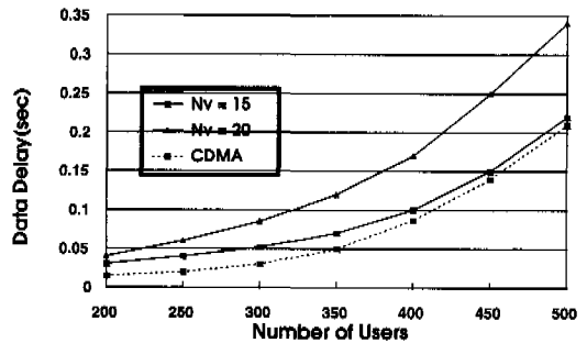
그림 12. 데이터전송 지연시간 (M=1Kbits, lambda d = 0.001msg/sec)
