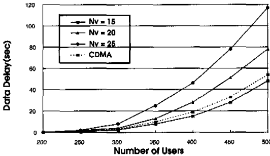
그림 13. 데이터전송 지연시간 (M=5Kbits, \lambda d = 0.001\text{msg/sec} )
