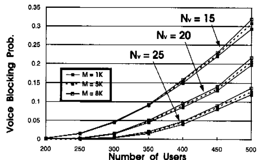
그림 4. D-TDMA 프로토콜에서 음성차단확률
