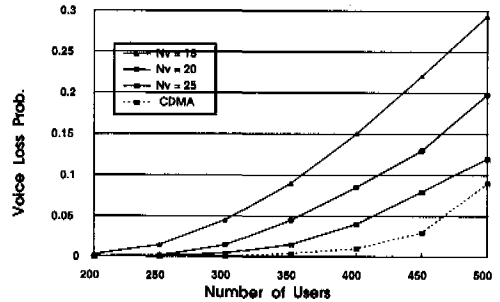
그림 11. CDMA 프로토콜에서 음성손실확률 (lambda d = 0.001msg/sec)
