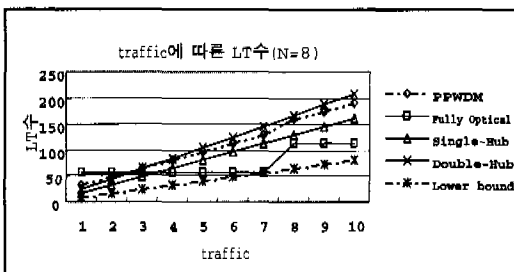
(d) 트래픽 부하에 따른 LT 수
