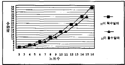
(b) 노드 수가 홀수와 짝수일 때의 비교
