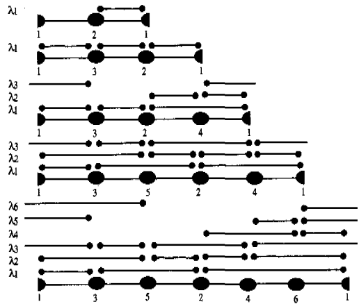
그림 5. 선형 구조에서 파장 할당 알고리즘에 따라 할당된 광 경로
