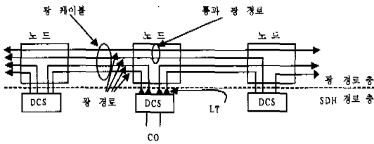
그림 1. 완전 광WDM 구조에서 OADM 노드의 기능
