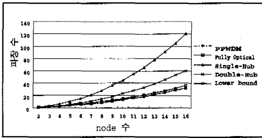
(a) 노드수에 따른 파장 수
