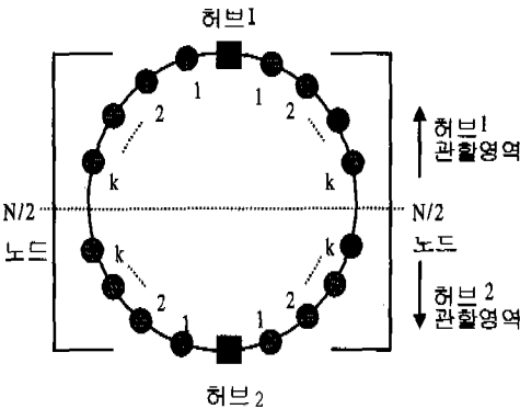
그림 2. DHWDM의 링 구조
