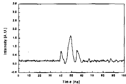
그림 6. 수신단에서 역 확산된 광 펄스 파형(Auto-Correlation)
