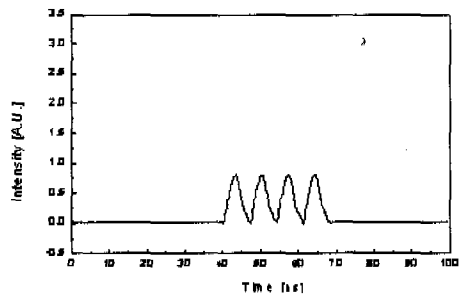
그림 5. 수신단에서 역 확산된 광 펄스 파형(cross-correlation)
