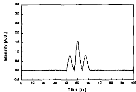
그림 4. 수신단에서 역 확산된 광 펄스 파형 (auto-correlation)
