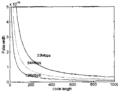
그림 14. 코드길이에 대한 레이저 광원의 선폭 변화
