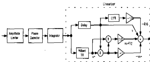
그림 2. RZ-SSB 수신기 구성도
