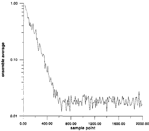
그림 5. SNR \infty dB인 경우의 수렴특성
