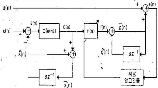
그림 2. 제한된 적응필터의 구조
