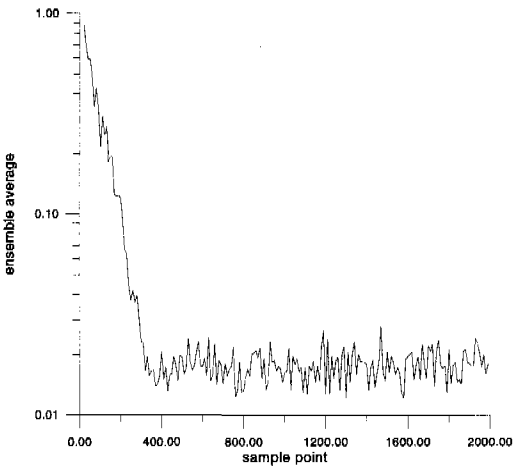
그림 6. SNR 30 dB인 경우의 Sign알고리즘 수렴특성
