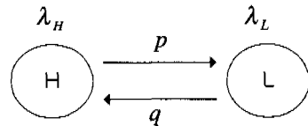
그림 2. MMPP model
