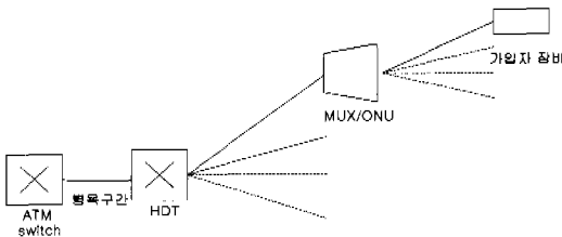
그림 1. 시스템 모델
