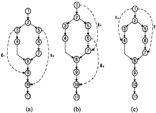
그림 3. 조건 분기들이 있는 경우의 중첩된 부그래프들
