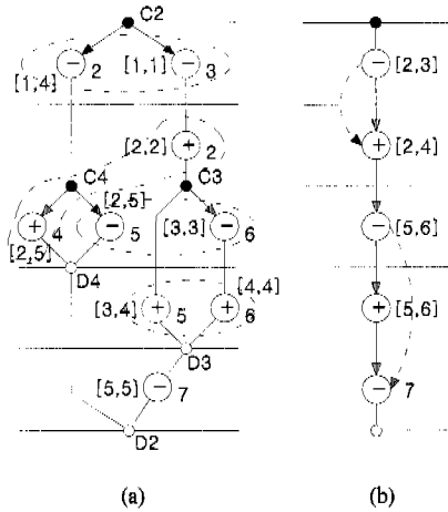
그림 6. 조건 분기들이 포함된 CDDG의 변환 a) 변환 과정 b) 변환된 CDDG
