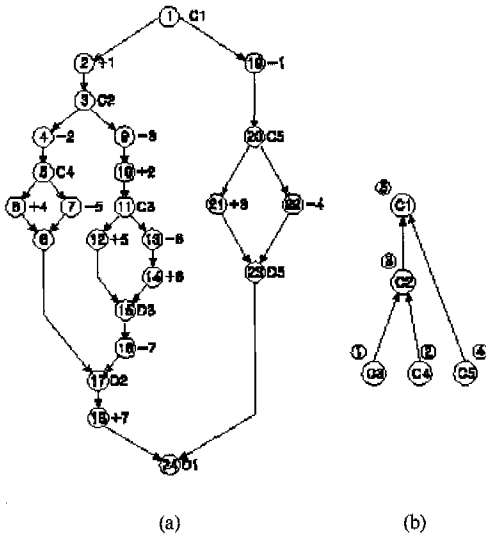
그림 5. 조건 순위 그래프의 구성 a) CDDG b) 조건 순위 그래프
