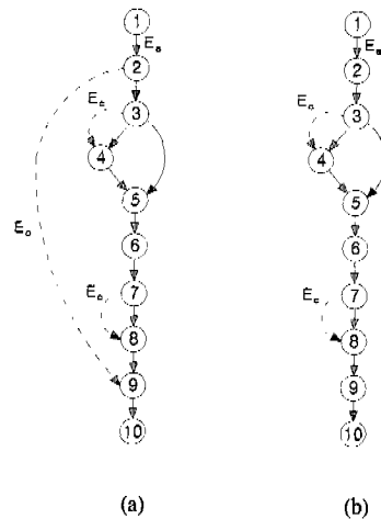
그림 2. 포함 관계를 갖는 부그래프의 제거 (a) 포함 관계를 갖는 부그래프 (b) (a)의 수정된 부그래프
