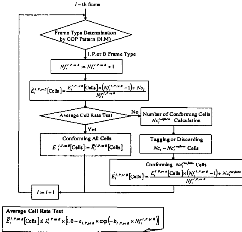
그림 8. Short-term 모니터링 순서도
