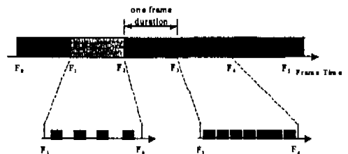
그림 2. VBR MPEG 인코더 셀 스트림 모델
