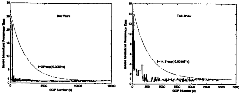
그림 10. 평균 패킷지연 변화
