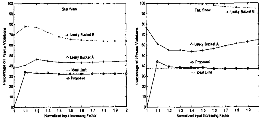
그림 13. I 프레임 셀의 부적합 비율 비교
