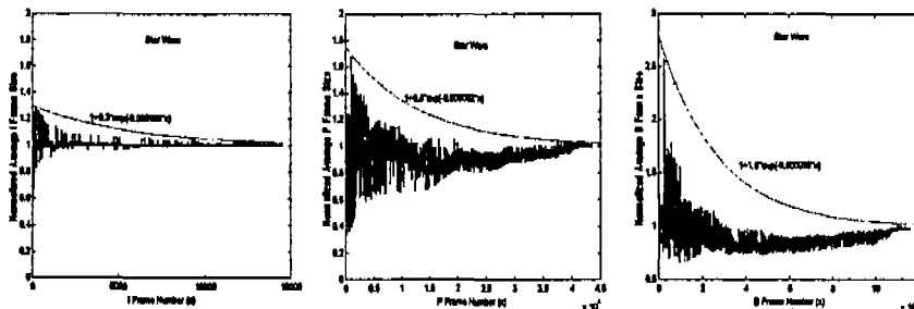
그림 11. 프레임 타임별 평균 셀 레이트 변화
