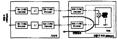
그림 4. 기지국에서의 반향 경로
