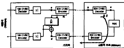
그림 7. 신호추정 필터 출력 \hat{x}(k) 를 참조신호로 사용하는 반향 제거기
