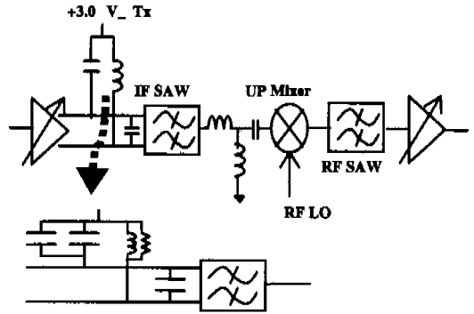
그림 3. TX IF SAW FILTER의 매칭
