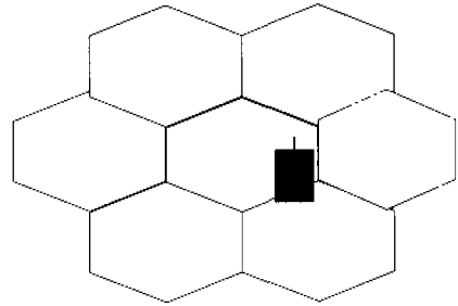
그림 5. 1계층 간섭 셀 모델
