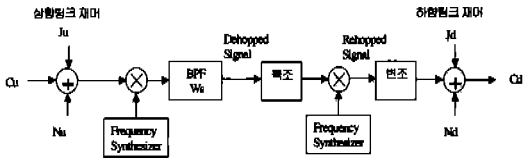
그림 4. SRT형 중계기 모델링 개념도
