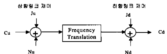
그림 1. BPT형 증계기 모델링 개념도
