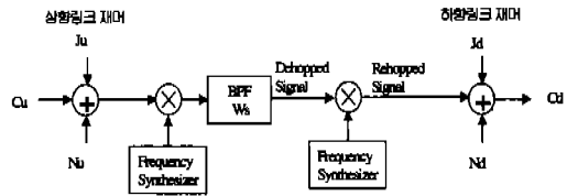
그림 3. DRT형 중계기 모델링 개념도
