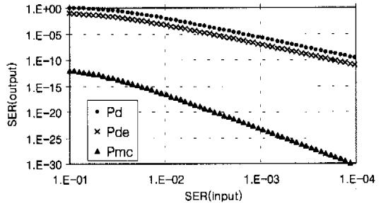
그림 3. Inner 복호 방법 2
