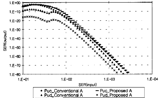
그림 5. 기존의 방법 A와 제안된 방법 A 비교 : Inner 부호 복호 방법 1 사용
