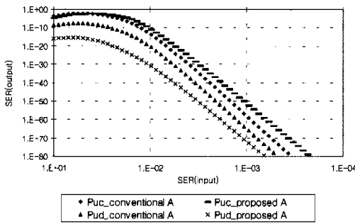
그림 8. 기존의 방법 A와 제안된 방법 A 비교 : Inner 부호 복호 방법 2 사용
