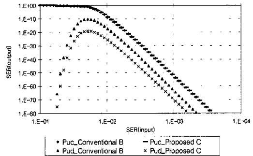
그림 6. 기존의 방법 B와 제안된 방법 C 비교 : Inner 부호 복호 방법 1 사용
