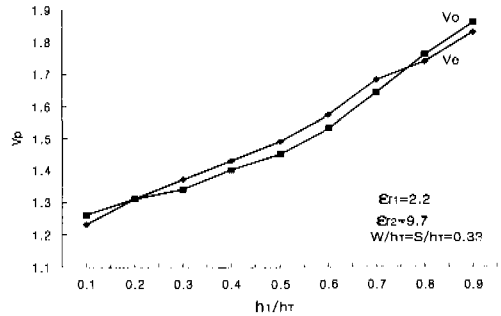
그림 2. 모드 위상속도
