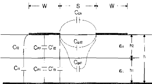
그림 1. 복합 유전체기판상에 결합 마이크로스트립 선로의 여러 가지 부유용량
