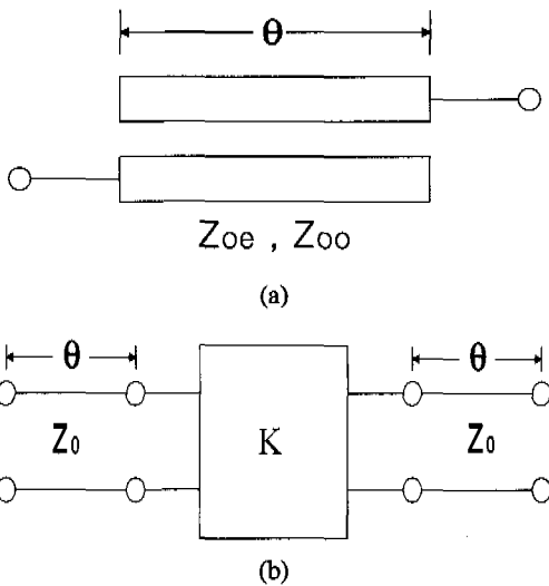
그림 5. (a) 결합 선로 (b) 등가회로
