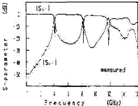
그림 9. 측정결과 [11] (단일기판)
