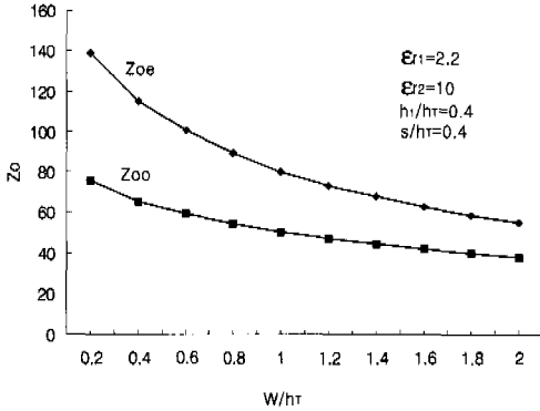
그림 4. 모드 임피던스
