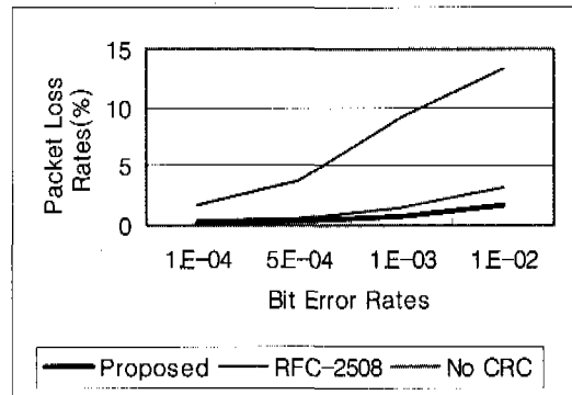
그림 7. BERs에 따른 패킷손실률의 변화
