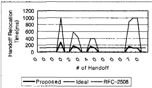
그림 9. 지연에 의한 Context 재 설정시간
