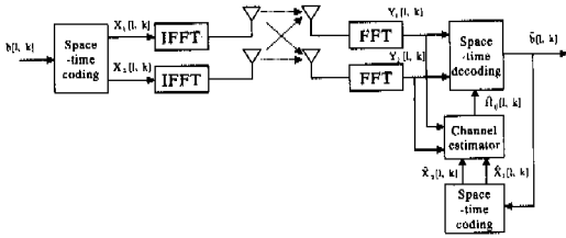
그림 1. Space-time coding을 이용하는 OFDM 시스템의 구성도
