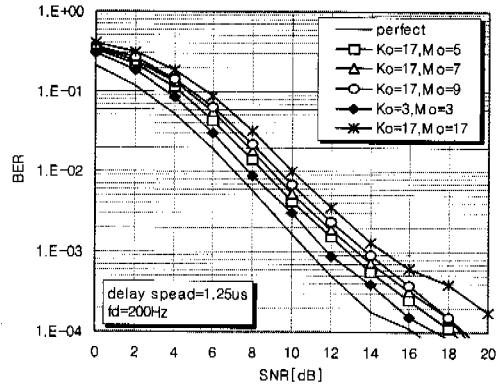
그림 5. BER 성능(rms delay spread=1.25us, fd=200Hz)
