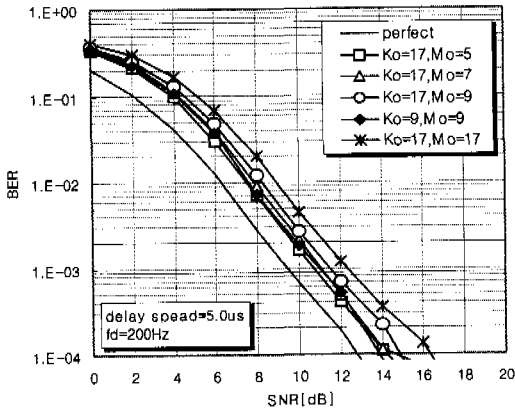
그림 7. BER 성능(rms delay spread=5us, fd=200Hz)
