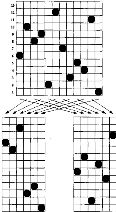
그림 3. 모듈라 소나배열의 Shuffling
