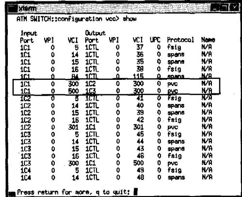
그림 16. ATM FORE switch에 설정된 PVC
