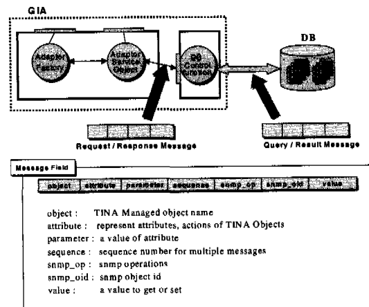
그림 9. Translation Message Format
