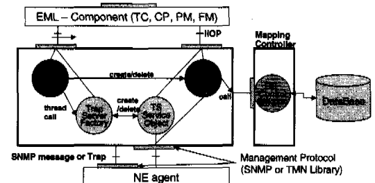
그림 2. Generic Interface Adaptor의 기능모델설계
