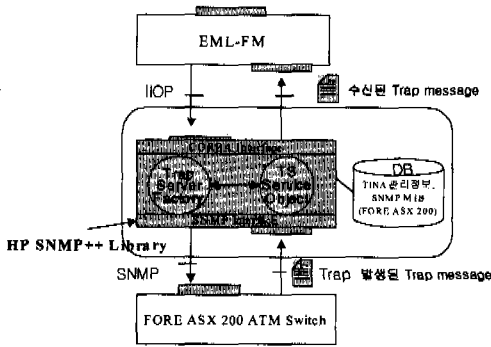
그림 17. 장애관리에 적용된 GIA
