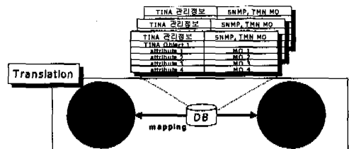
그림 4. Message Translation
