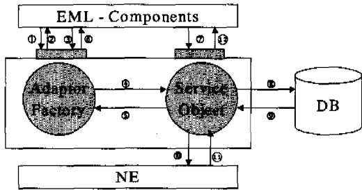
그림 10. GIA의 동작절차
