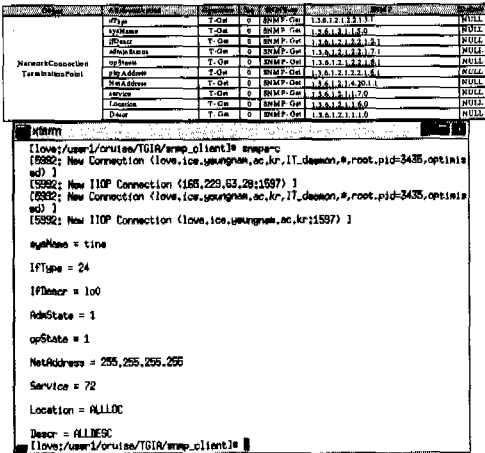
그림 14. NetworkTerminationPoint의 Template추정결과
