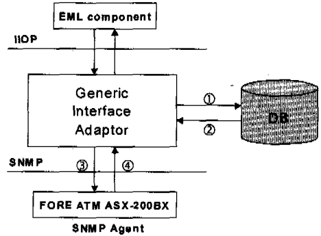
그림 19. Operation 실행순서
