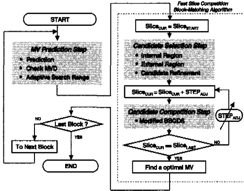
그림 12. HSR방식의 흐름도
