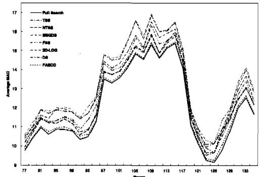
그림 15. 프레임 측에 대한 평균 MAD (Football2 (frame77~135))
