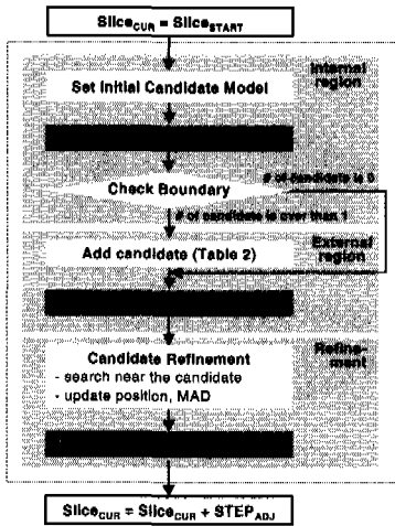
그림 13. CCS의 흐름도
