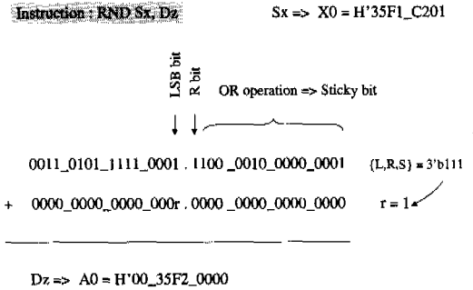
그림 5. YS-RDSP의 라운딩 연산
