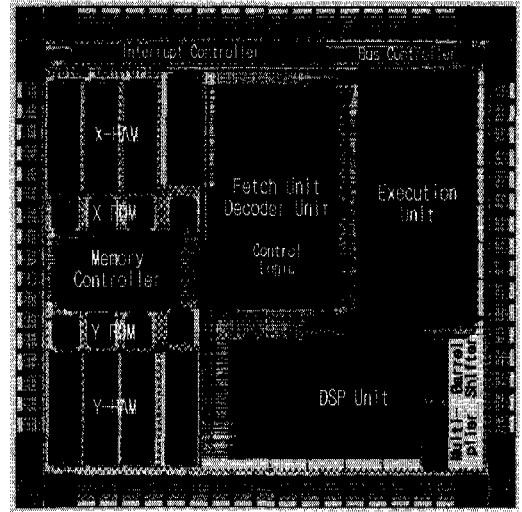
그림 12. YS-RDSP 레이아웃
