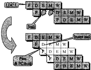
그림 9. Flush 신호 제어의 예
