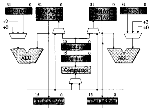
그림 3. 모듈로 주소 생성기
