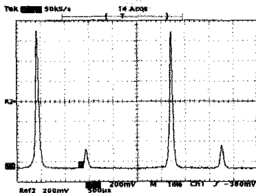
그림 5. 시간 영역에서 패브리 퍼롯 간섭계를 통해 나타난 브릴루앙 신호
