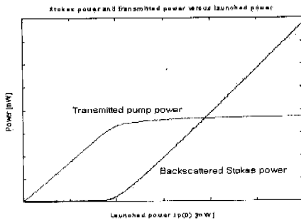
그림 3. 입력 펌프 함수 I_p(0) 에 대한 전송된 펌프 신호와 후방 산란된 Stokes 신호
