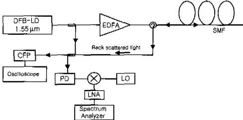
그림 4. SBS 신호 측정을 위한 실험 장치
