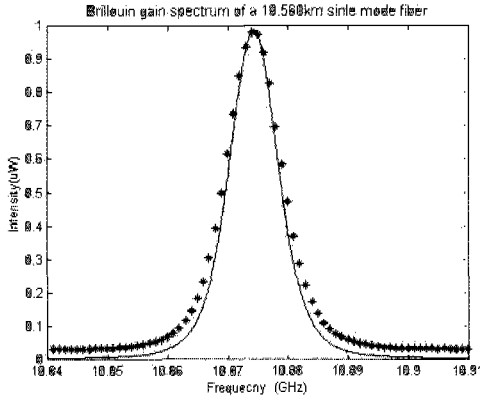
그림 11. 입력 파워가 4.406mW, 초기 Stokes 파워가 0.3414 \mu W인 경우의 BGS
