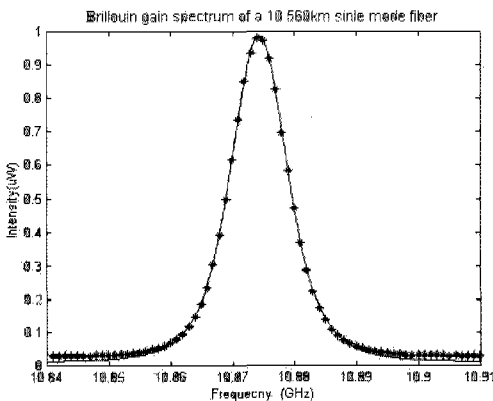
그림 13. 입력 파워가 4.406mW, 초기 Stokes 파워가 1.564 \mu W인 경우의 BGS
