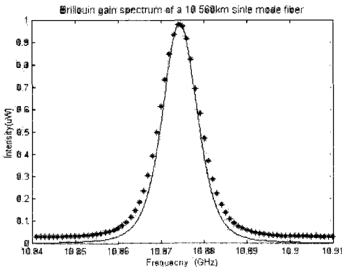
그림 12. 입력 파워가 7.943mW, 초기 Stokes 파워가 0.3414 \mu W인 경우의 BGS
