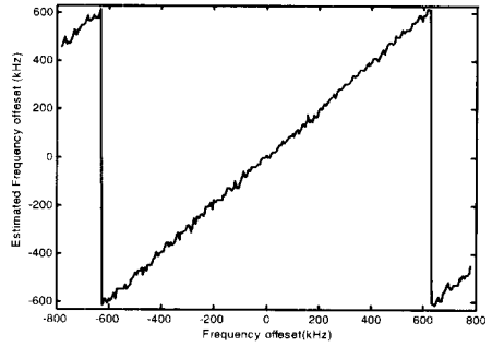
(b) 그림 6. 초기 반송파 주파수 옵셋의 추정범위
