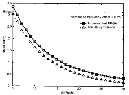
그림 9. 미세 반송파 주파수 옵셋 추정에 대한 시뮬레이션 결과와 FPGA 구현 결과의 RMSE 성능 비교
