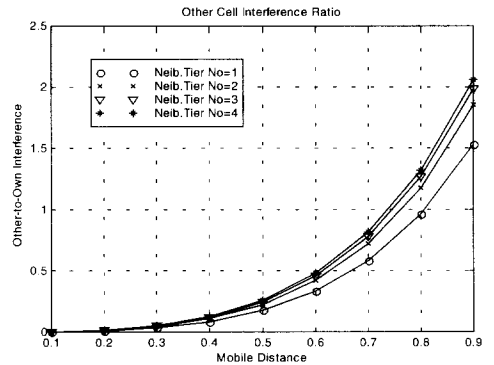
그림 6. 셀 환경에 정규화 한 단말의 거리에 따른 타셀 간섭 계수.
