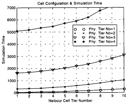
그림 10. 셀 구성에 따른 시뮬레이션 소요 시간
