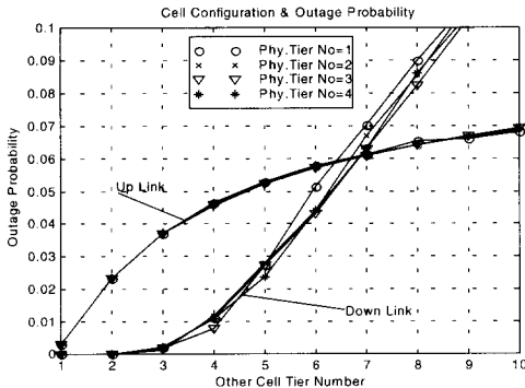
그림 4. 셀 구성과 Outage 확률
