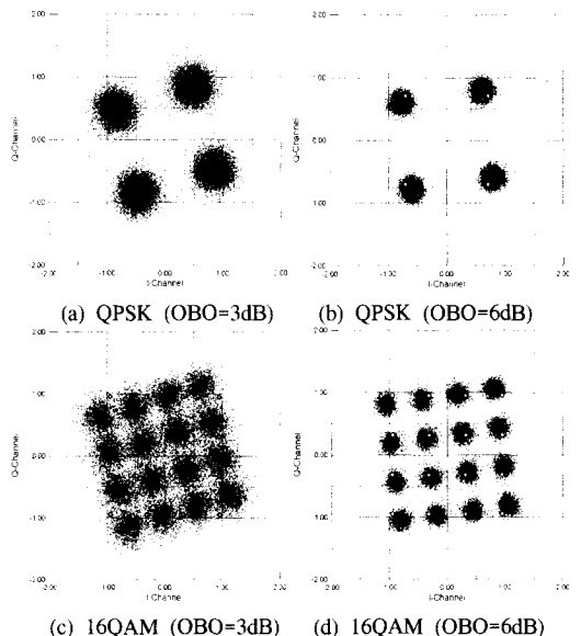
그림5. TWTA의 OBO 값에 따른 신호 정상도 Fig. 5. Signal constellation to OBO value of TWTA
