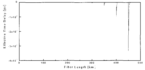
(c) 10 스패 광섬유 링크의 경우 (500 km)
