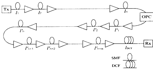
그림 4. OPC와 DCF를 혼합한 MI 보상구조
