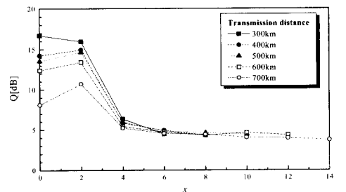
그림 6. x 값에 대한 전송거리별 성능 ( 40 Gb/s, SMF )
