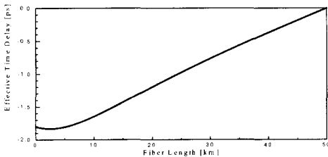
(a) 단일 스패 광섬유의 경우
