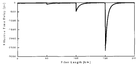
(b) 4 스패 광섬유 링크의 경우 (200 km)
