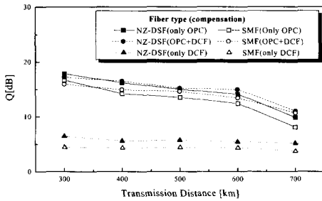
그림 7. SMF와 NZ-DSF에 대한 MI 보상성능 비교 (40 Gb/s)
