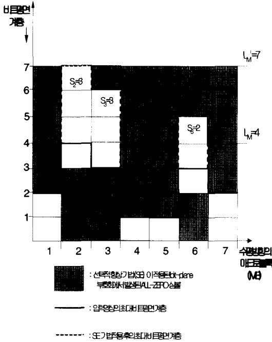
그림 3. SE 기법 적용후의 FGS 비트평면 구조도
