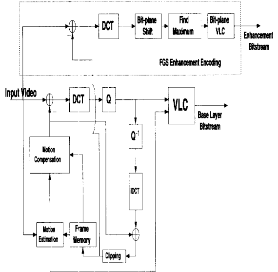
그림 1. 표준 MPEG-4 FGS 부호기의 구조도
