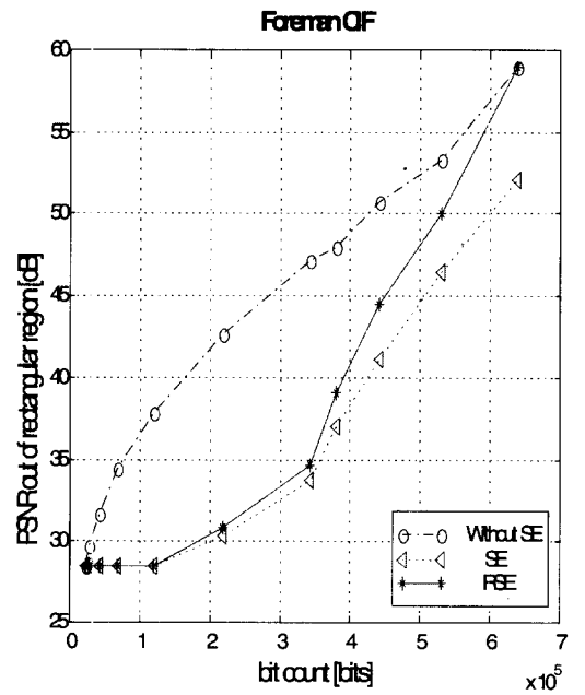
그림 11. Foreman CIF 영상 1번째 화면(I-화면)에서 비중요영역의 PSNR 성능 비교
