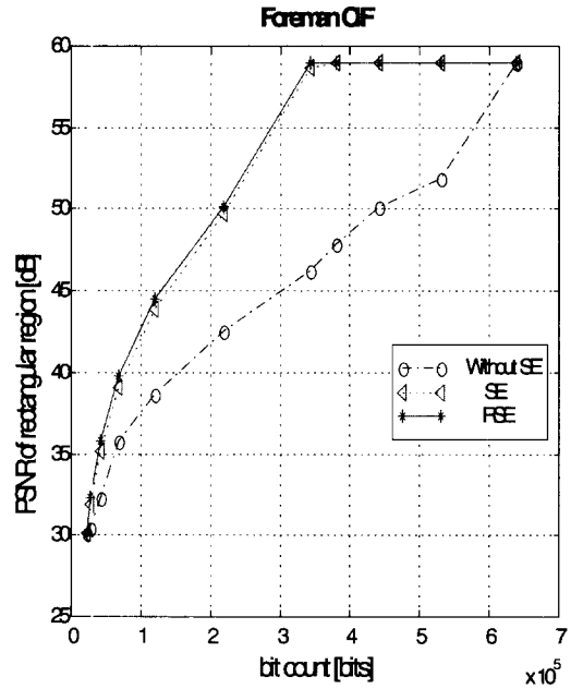
그림 10. Foreman CIF 영상 1번째 화면(I-화면)에서 중요영역의 PSNR 성능 비교
