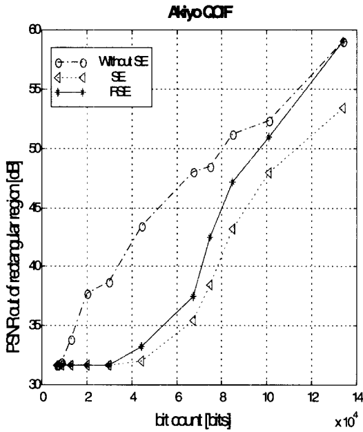
그림 8. Akiyo QCIF 영상 1번째 화면(I-화면)에서 비중요영역의 PSNR 성능 비교
