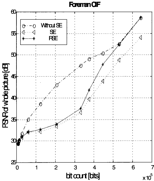
그림 12. Foreman CIF 영상 3번째 화면(P-화면)에서 화면 전체의 PSNR 성능 비교
