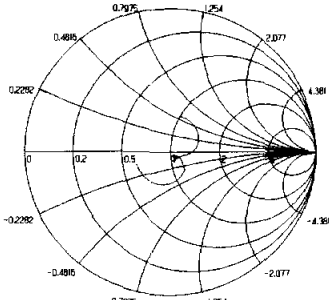
(a) 90° 위상 지연
