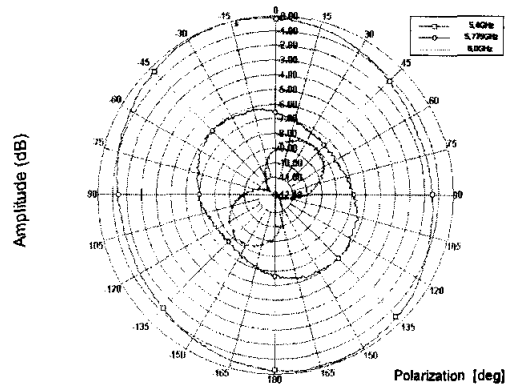
(a) 90° 위상지연
