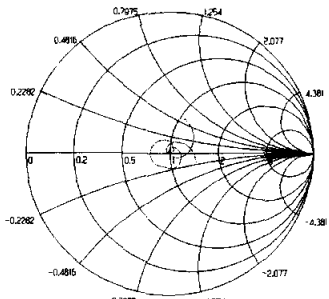
(b) 45° 위상 지연
