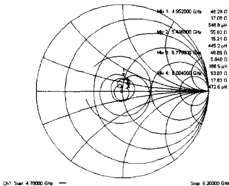
(b) 45° 위상지연
