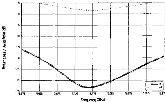
그림 4. 단일 패치 안테나 시뮬레이션 결과
