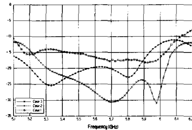
(a) 반사손실 특성
