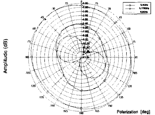
(b) 45° 위상지연
