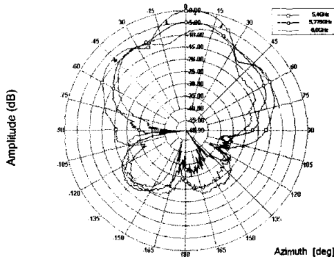
(b) 45°위상지연
