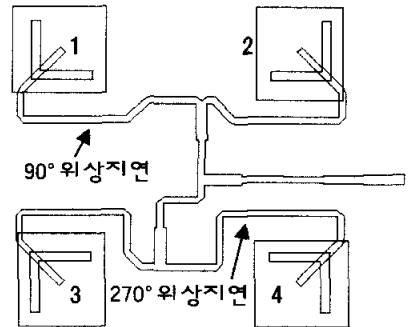
그림 5. 시퀀셜 로테이션 배열
