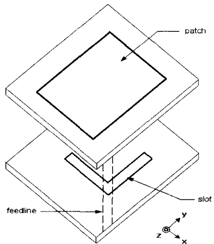
그림 1. L자형 개구 결합 원형편파 패치 안테나 구조
