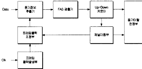
그림 7. 제안한 동기이탈 검출 기능 블록도
