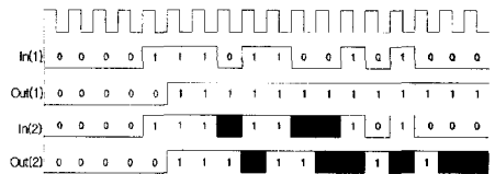
그림 3. MLS 프레임 검출
