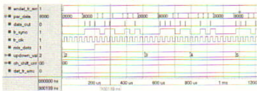
(a) 동기비트가 첫 번째 채널에 있을 경우
