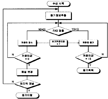
그림 8. 제안한 동기이탈 검출 절차
