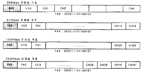
그림 2. 프레임 구조
