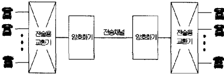
그림 1. EUROCOM 통신시스템
