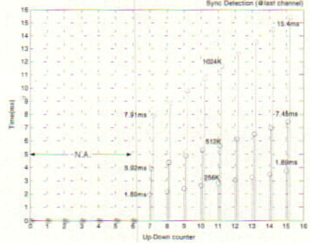
그림 10. Up-Down 카운터값에 의한 동기 검출 시간
