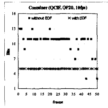
그림 8. 화면당 발생하는 화면 종료 신호에 대한 기존 방식과 EOF 신호로 하는 제안 방식에서의 비트 수
