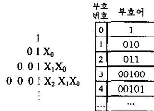
그림4. H.264 Exp-Golomb 부호어 구조 형태
