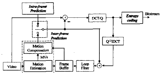
그림 1. H.264 동영상 압축 부호화 블록도
