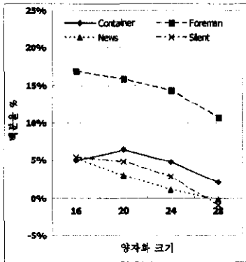
그림 12. RUN, MB_type 구문 요소를 독립적으로 부호화하던 기존 방식 대비 제안한 구문 요소로 부호화한 제안 방식의 전체 평균 비트 감소율
