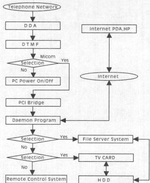
그림 7 Teleremote 시스템의 순서도
