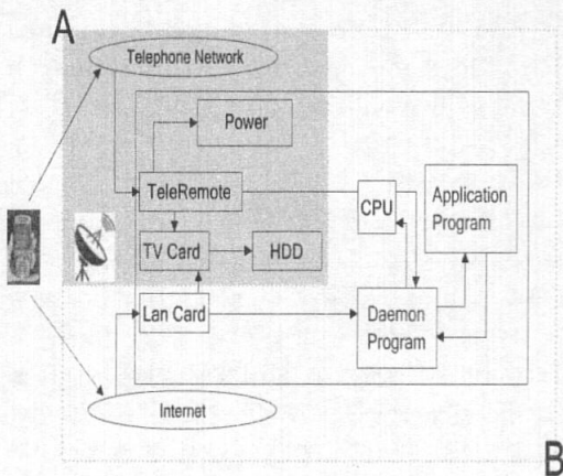
그림 6. TeleRemote 제어 시스템 설계 블록도
