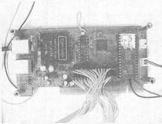
그림 8. TeleRemote system 제작한 보드
