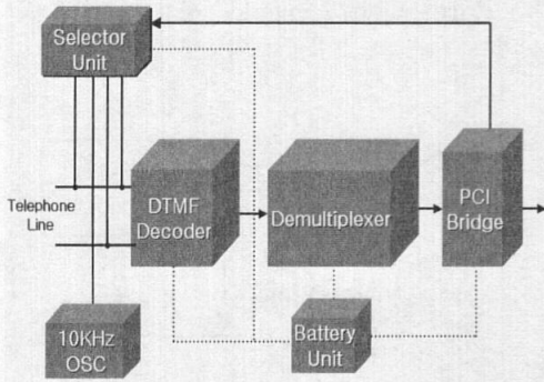
그림 2. 일반 단순형 제어 장치 블록
