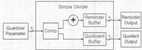
그림 11. Simple Divider 모듈의 구조
