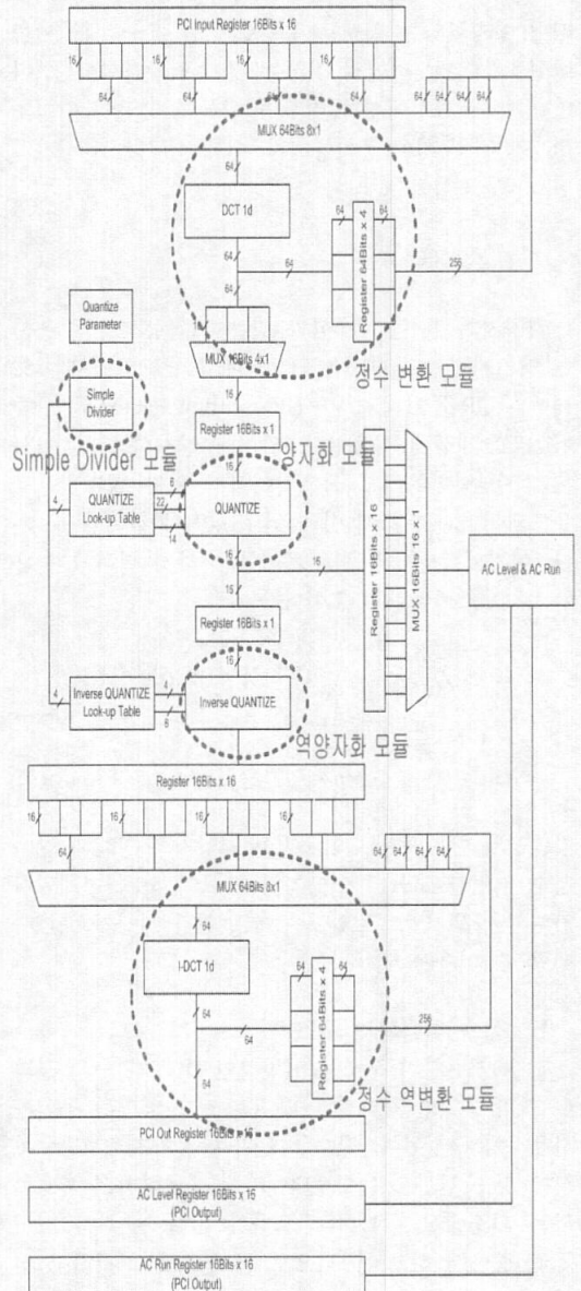
그림 5. 전체 모듈 블록도
