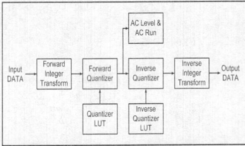
그림 4. 영상 데이터의 흐름도
