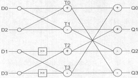
그림 9. IDCT-1d의 구조
