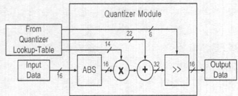
그림 8. 양자화 모듈의 구조
