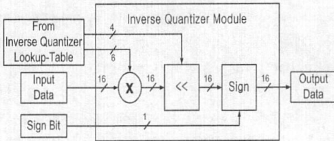
그림 10. 역양자화 모듈의 구조
