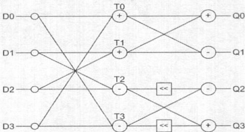
그림 6. DCT-1d의 구조
